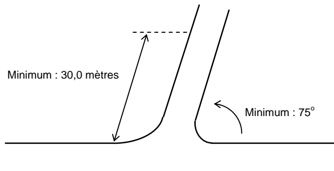
FIGURE 5.4 : ANGLE ENTRE DEUX INTERSECTIONS
